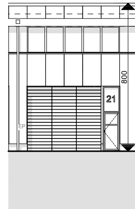
Façade Sud 1:200
